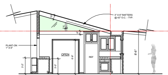
ELEV. K
