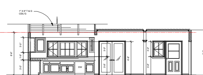
ELEV. H
