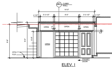
ELEV. I
