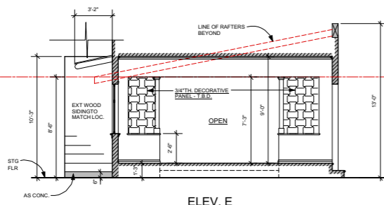
ELEV. E
