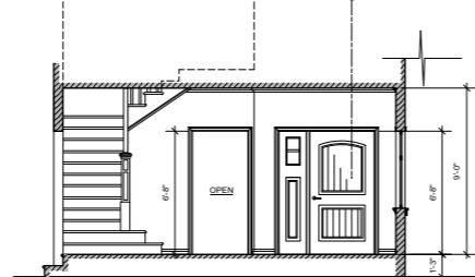
ELEV. F
