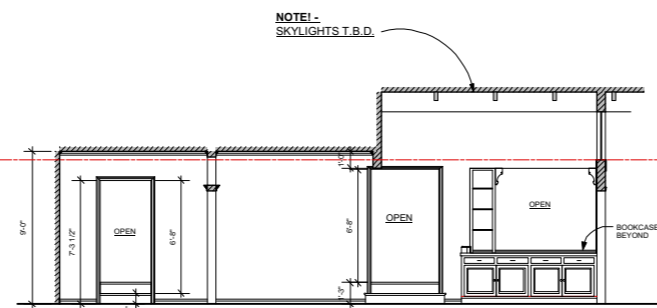
ELEV. J
