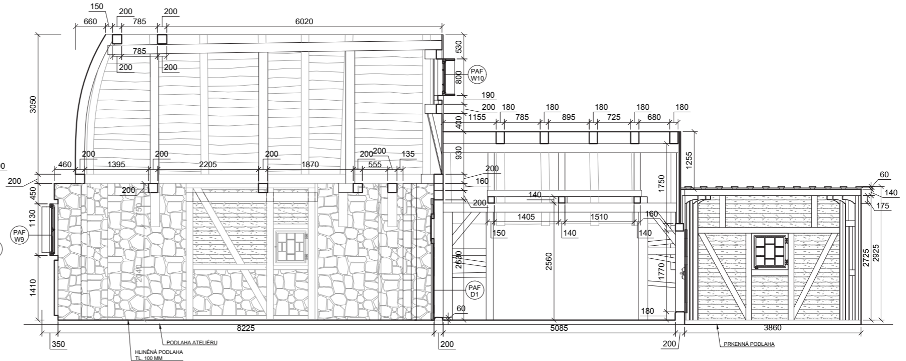
ŘEZ BB_1:50 SECTION BB_1:50
