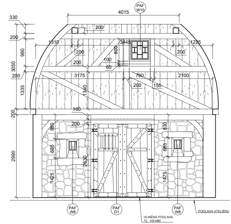
POHLED C_1:50 ELEVATION C_1:50
