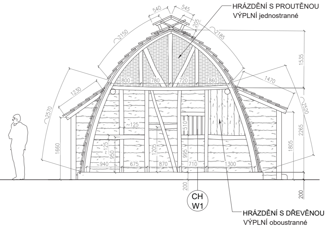
POHLED ZADNÍ, M 1:50
