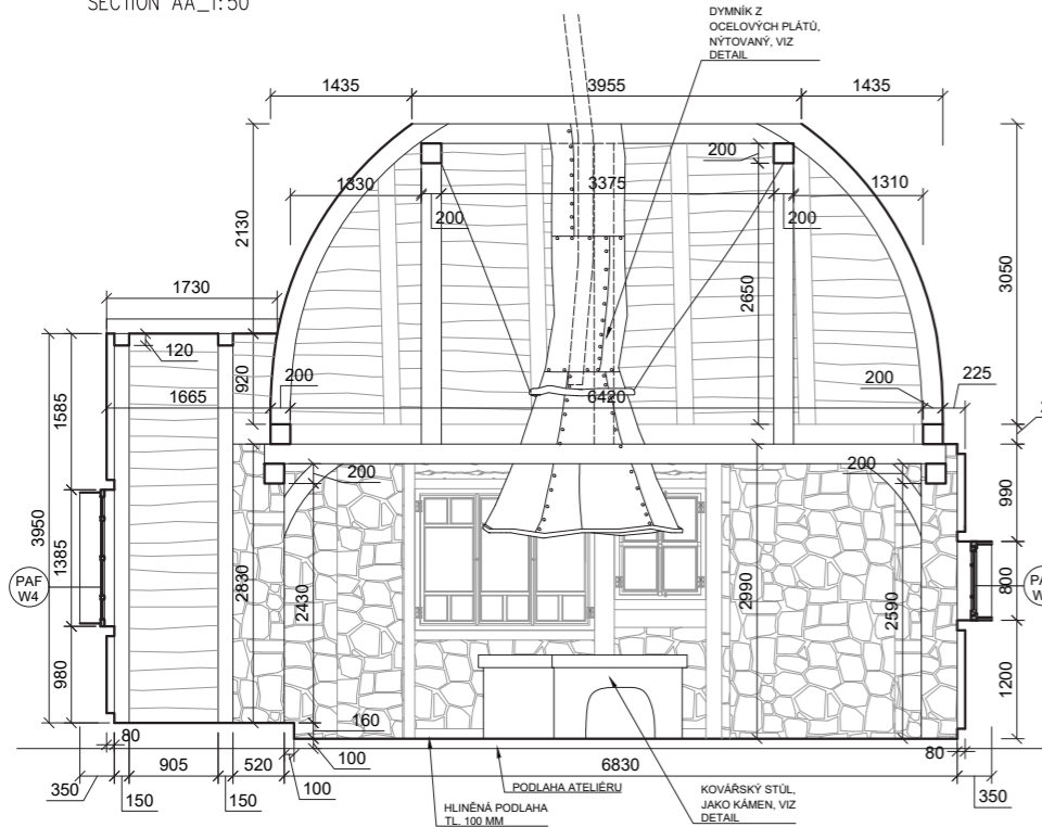
ŘEZ AA_1:50 SECTION AA_1:50
