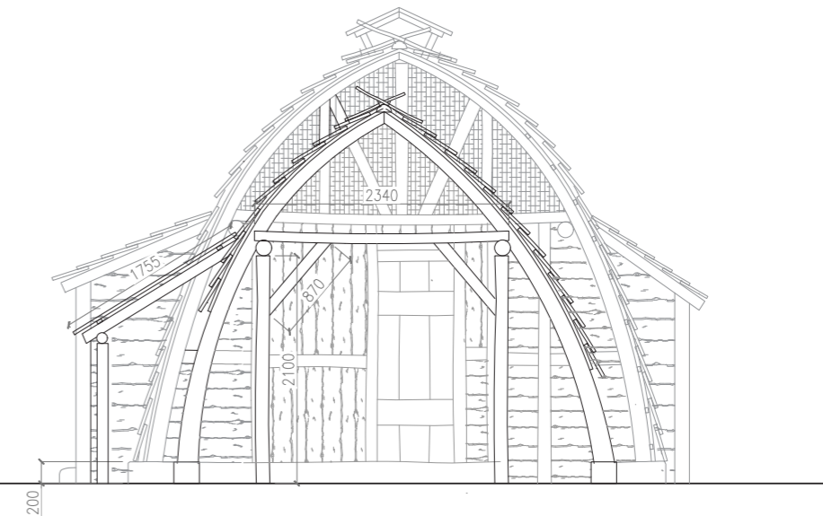
POHLED ZADNÍ, M 1:50
