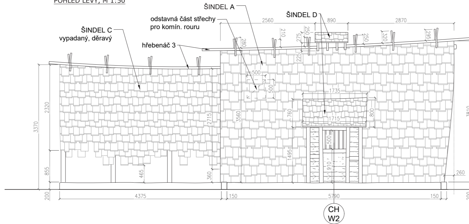
POHLED LEVÝ, M 1:50
