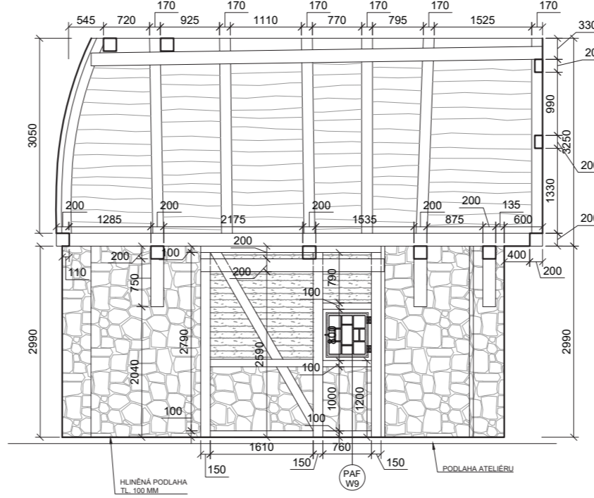
POHLED B_1:50 ELEVATION B_1:50
