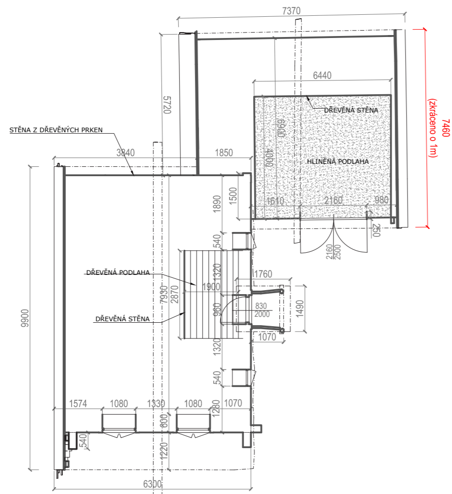
PŮDORYS, M 1:100
