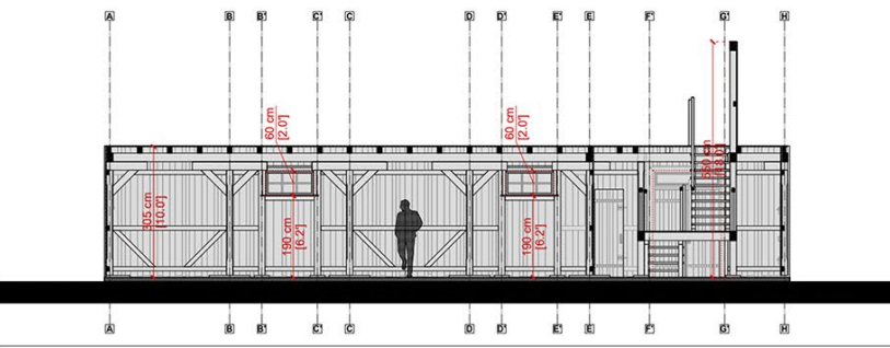
Longitudinal section 2 / Sc. 1:50
