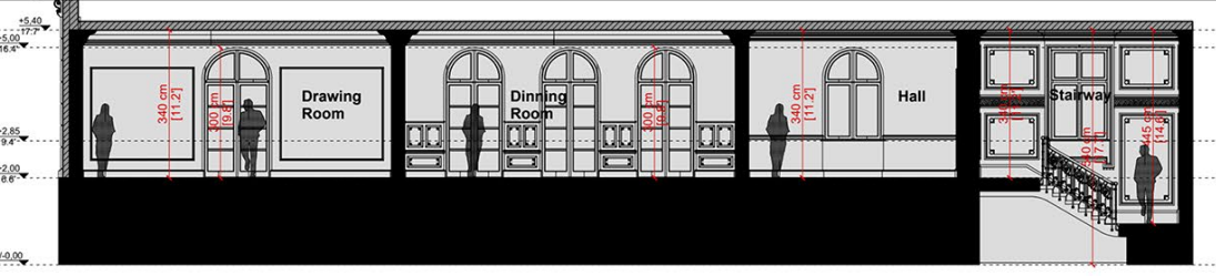
Longitudinal section / Sc. 1:50
