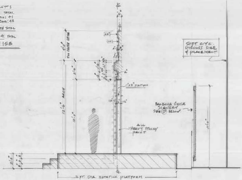
B SECTION A-B
