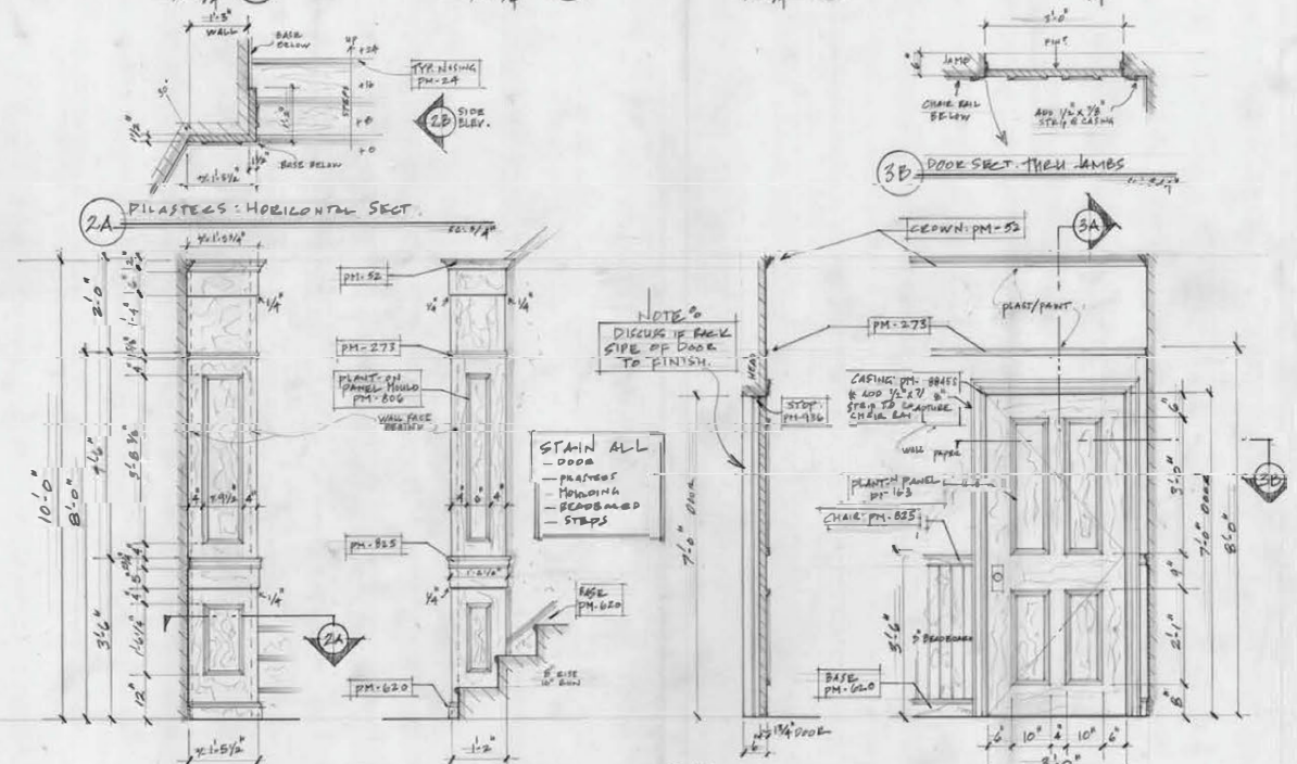
DET. 2 PILASTER: FRONT VIEW DET. 2B PILASTER: SIDE VIEW DET. 3A HEAD SECT. DOOR DET. 3 DOOR
