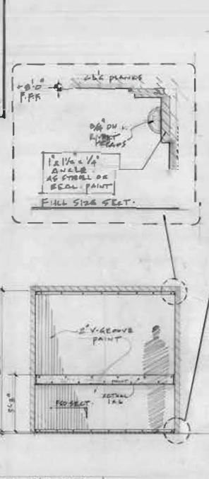
(D) INT. ELEVATION 1/2" = 10'-0"
