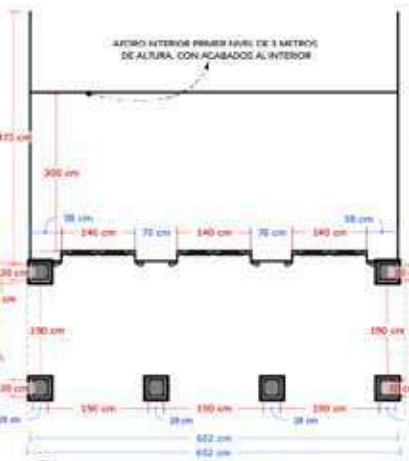
6 PLANTA PRIMER NIVEL CASA 9 - ZONA 12 ESC. 1:50
