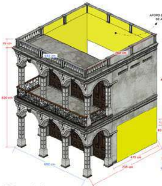
5 AXONOMETRIA A CASA 9 - ZONA 12 ESC. 1:40
