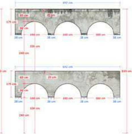
4 ALZADO FRONTAL ARCADEA CASA 9 - ZONA 12 ESC. 1:30
