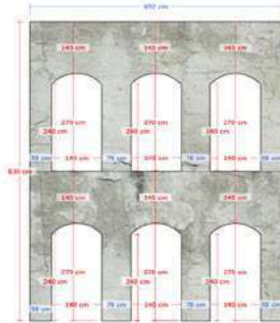
2 ALZADO FRONTAL BASTIDOR CASA 9 - ZONA 12 ESC. 1:30
