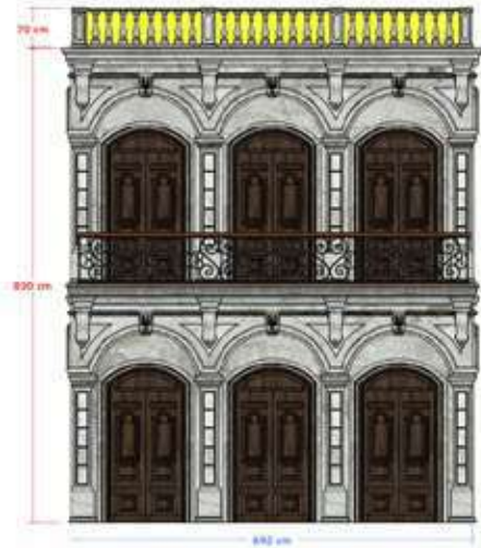
1 ALZADO FRONTAL CASA 9 - ZONA 12 ESC. 1:30
