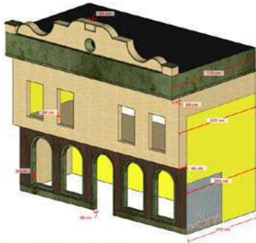
5 AXONOMETRIA BASTIDOR ZONA 12 - CASA 13 PIETRO CRESPI ESC: 1/75
