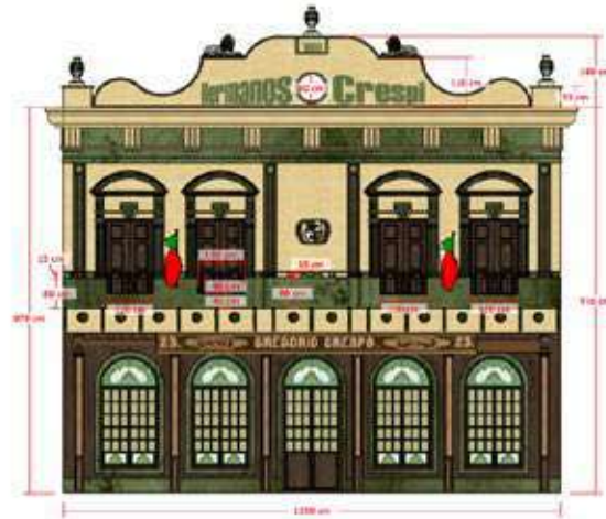
2 ALZADO FRONTAL ZONA 12 - CASA 13 PIETRO CRESPI ESC: 1/75
