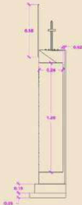
CORTE DETALLE 1
