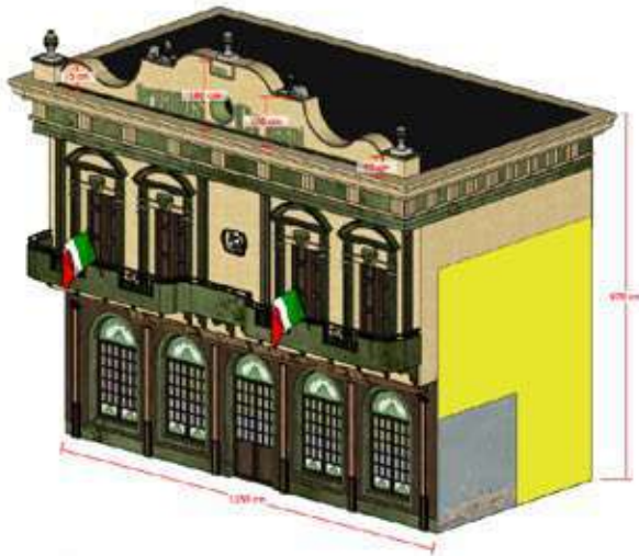
1 AXONOMETRIA ZONA 12 - CASA 13 PIETRO CRESPI ESC: 1/75
