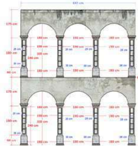
3 ALZADO FRONTAL ARCADEA Y COLUMNAS CASA 9 - ZONA 12 ESC. 1:30
