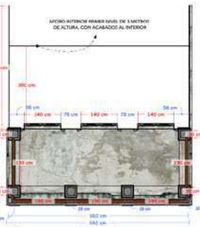
7 PLANTA SEGUNDO NIVEL CASA 9 - ZONA 12 ESC. 1:50
