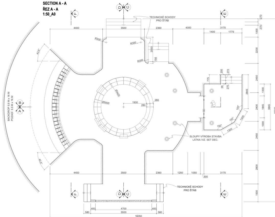
PLAN PŮDORYS 1:50_A0
