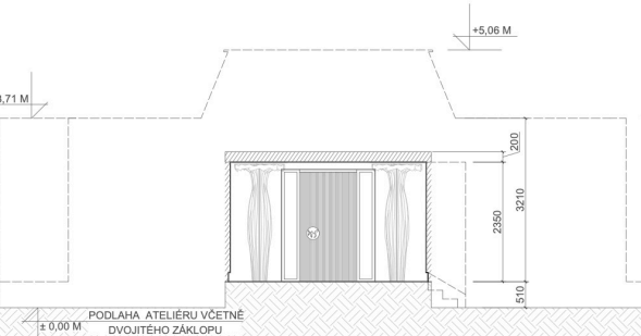
SECTION E - E REZ E - E 1:50_A0
