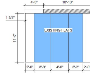
E E WALL ELEV Scale: 1/4" = 1'-0"
