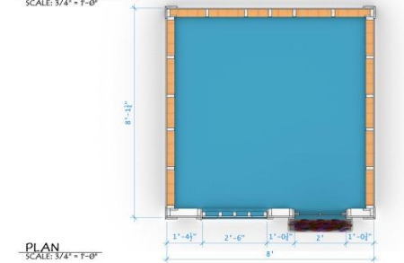
PLAN SCALE: 3/4" = 1'-0"
